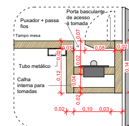
DET.06 | PASSAFIOS + CALHA ESC: 1:5
