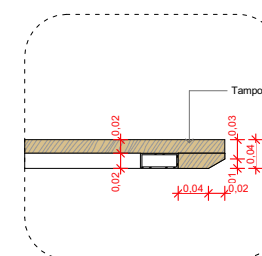
DET.05 | CHANFRO BANCADA ESC: 1:5
