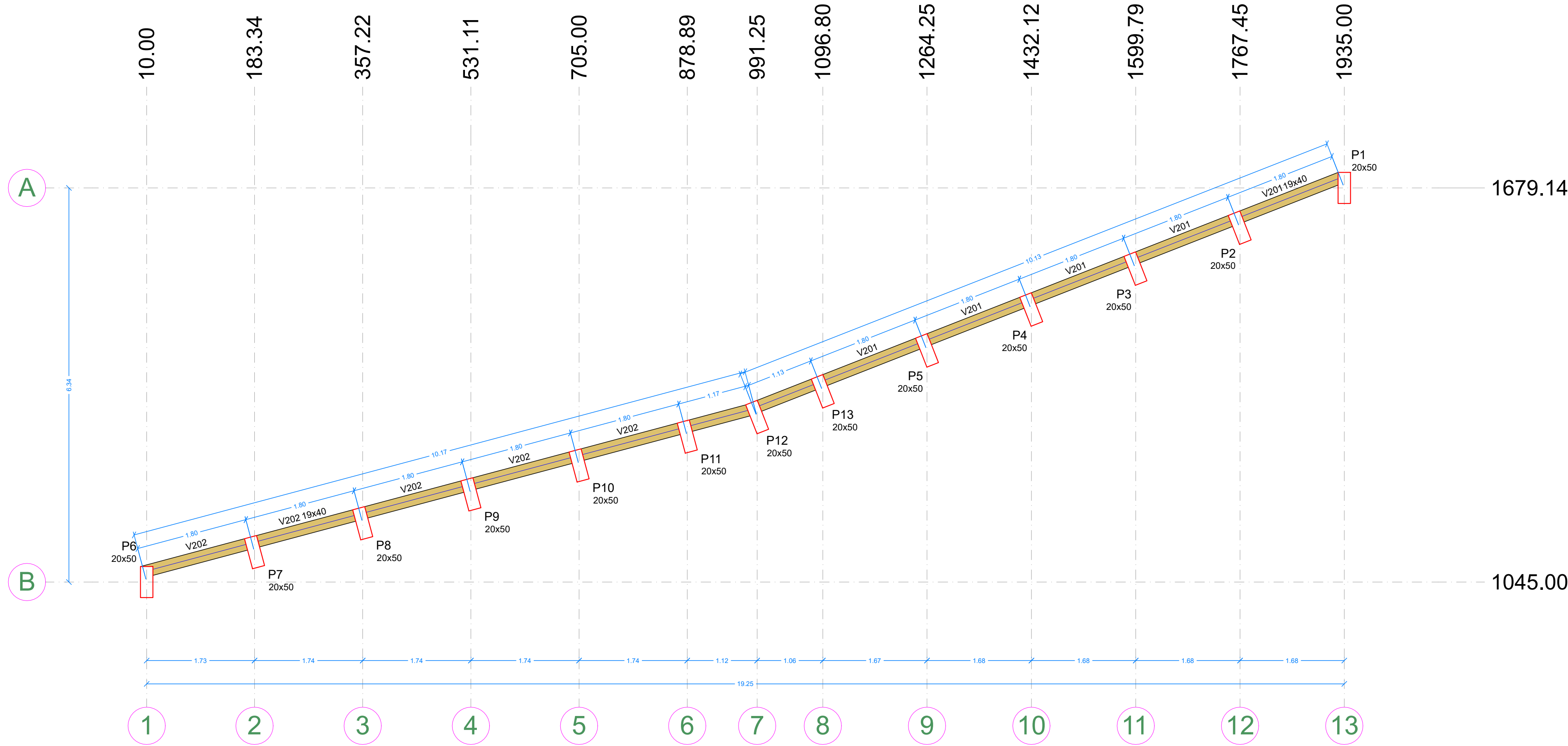
FORMA DO PAVIMENTO RESPALDO -300 ESCALA 1:50
