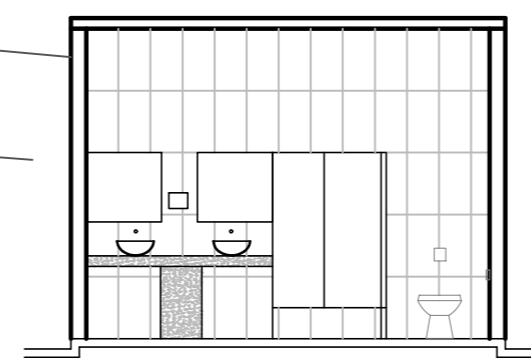
DETALHE BANHEIROS
